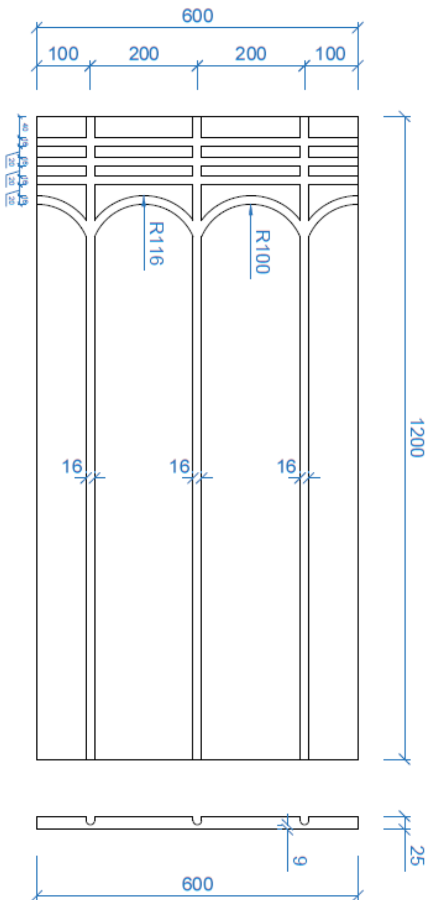
TYCROC UHP20 TECHNICAL DIMENSIONS
