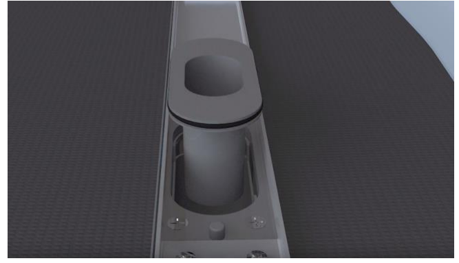
12. Laita kolmas kumitiiviste hajulukon (nro 2) vastaavaan uraan ja asenna osat lattiakaivon runkoon (nro 6). Täytä ruostumattomasta teräksestä valmistettu lattiakaivon kourun sisusta lattialaattalla (liimaamalla) ja laita se paikalleen kouruun
